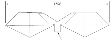
Anschlussmaß d=80mm
